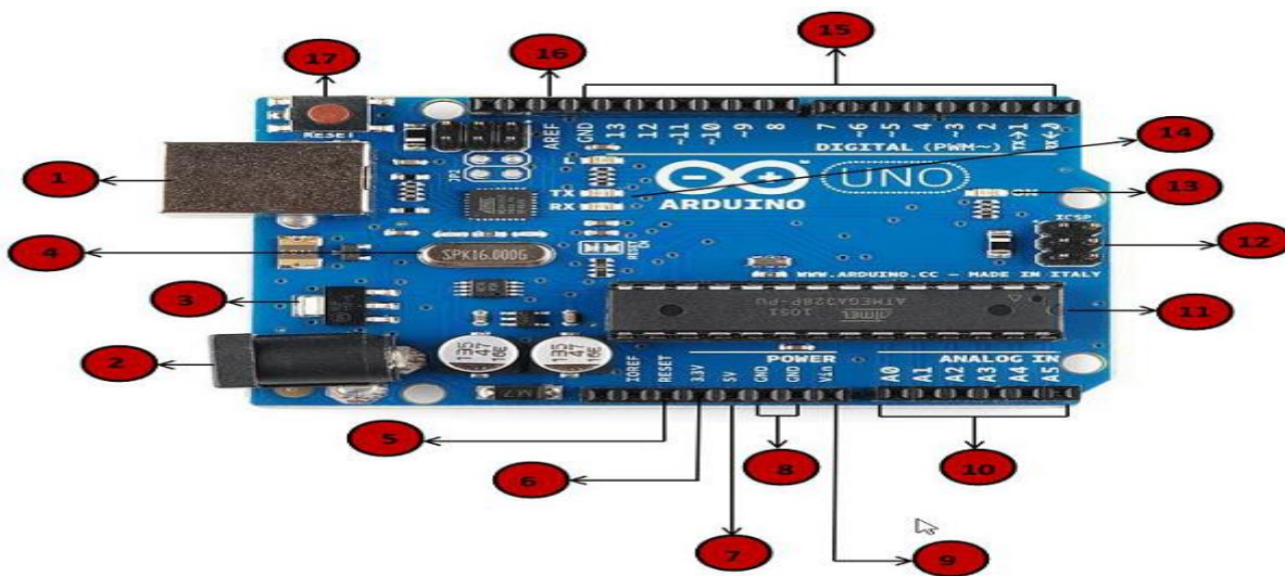
Fig2: Arduino Uno
