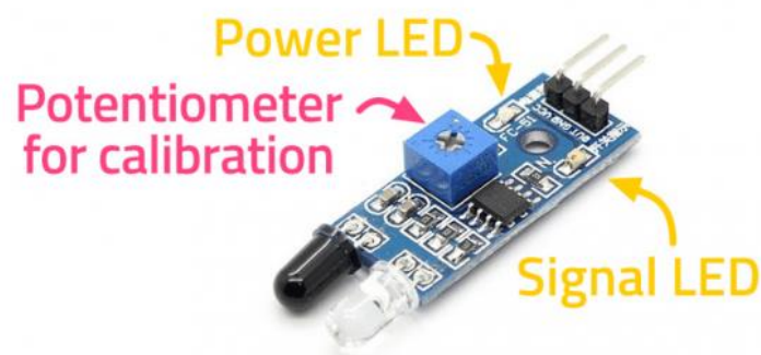
Fig4: IR Module
